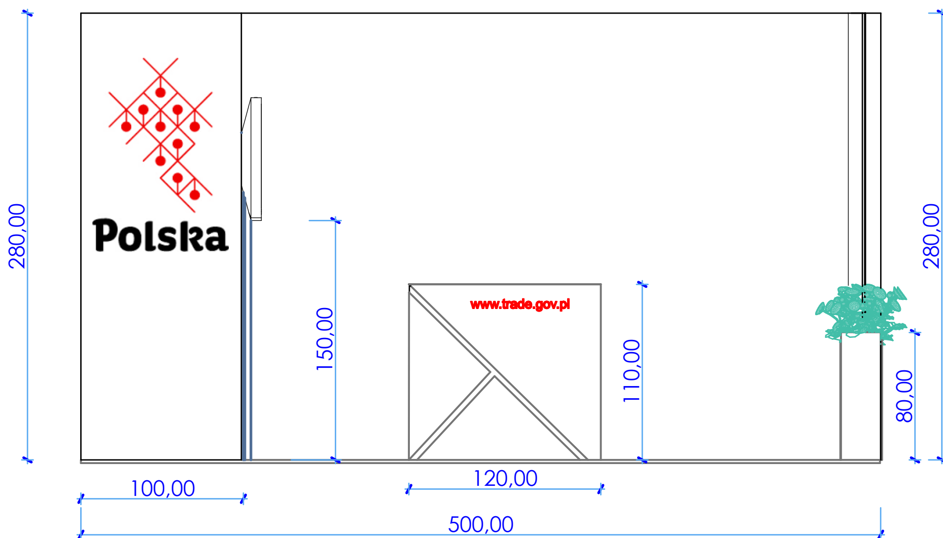
PRZEKRÓJ A-A
